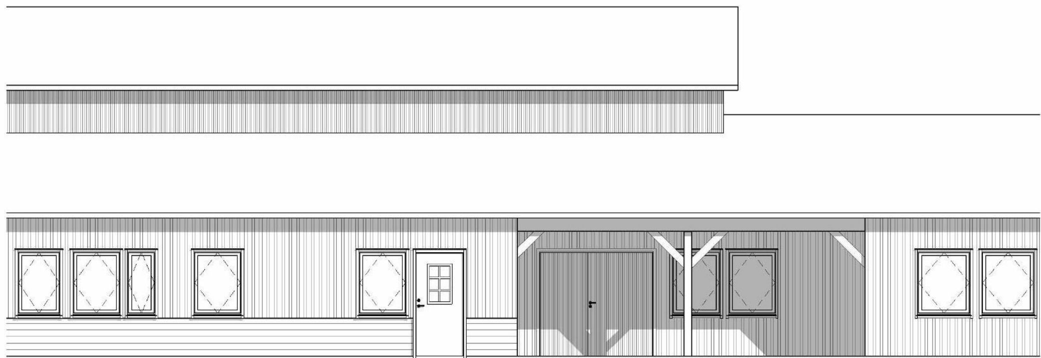
Fasade Sørøst
